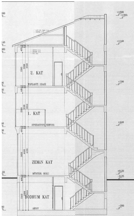
A.A KESİTİ ÖLÇEK:1/50
