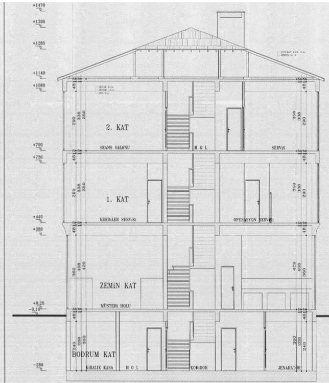
B.B KESİTİ ÖLÇEK:1/50
