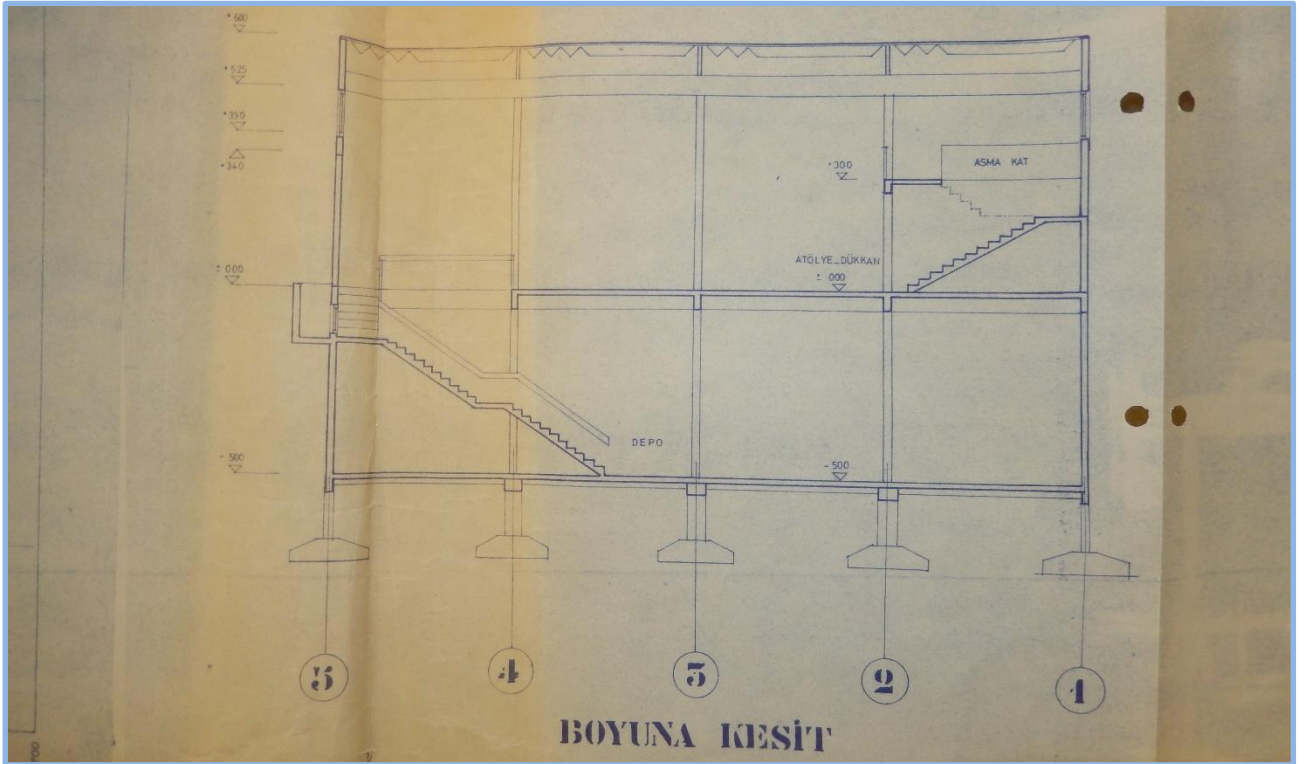
Boyuna Kesit
