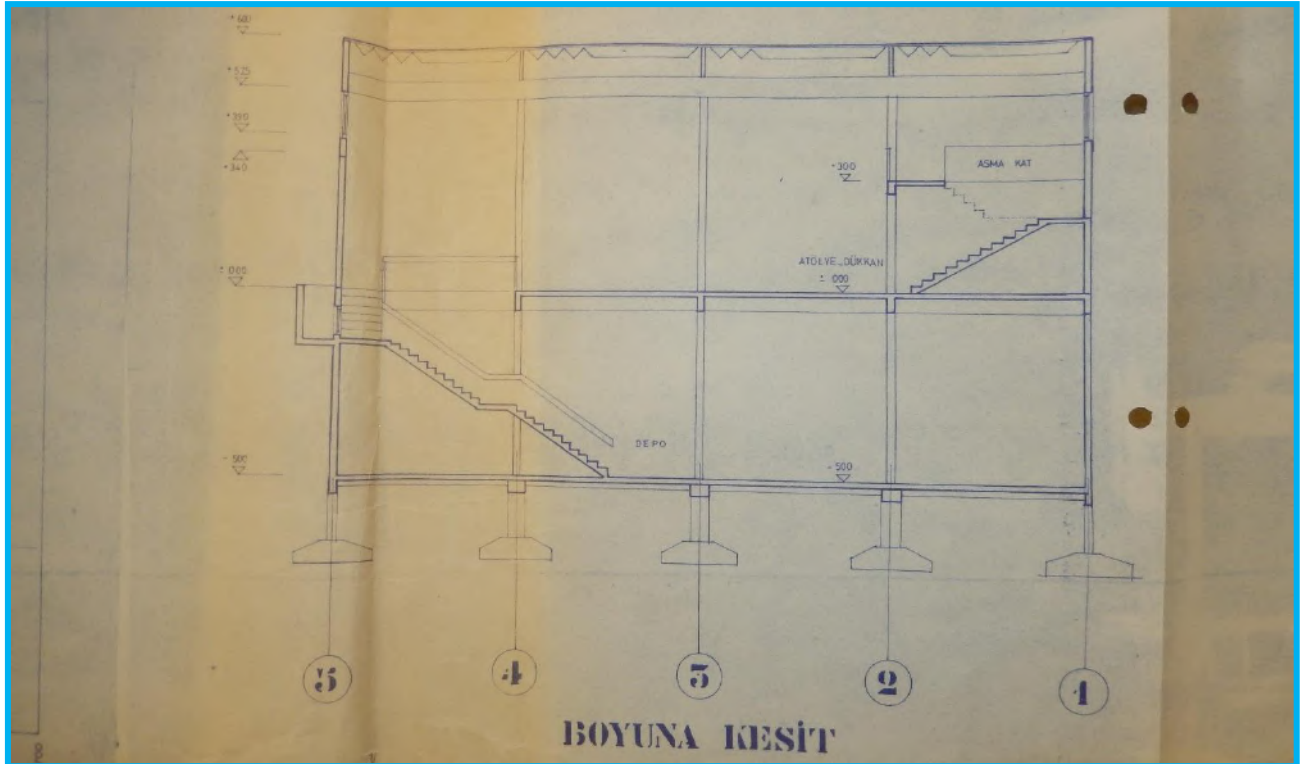
Boyuna Kesit
