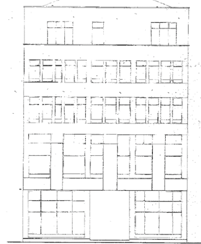
ARKA CEPHE 0 1/50
